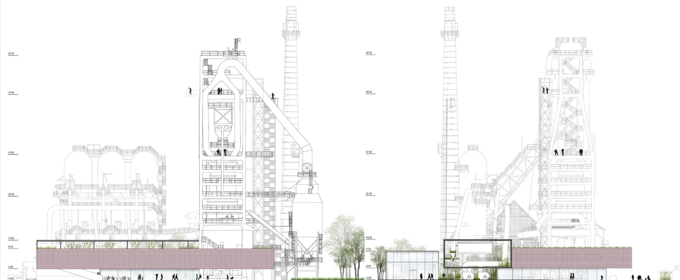
Elevacja Zachodnia / M1:250
